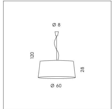
SP 7/505 1 x max 77W E27 CE IP20 ▽
