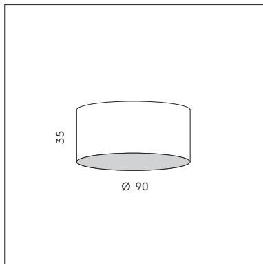
LS P/503-L 3 x max 77W E27 CE IP20 ▽
