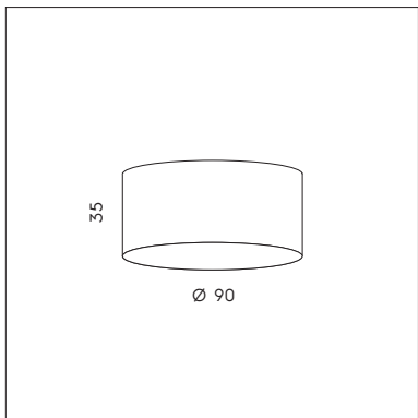
LS P/503 3 x max 77W E27 CE IP20 ▽
