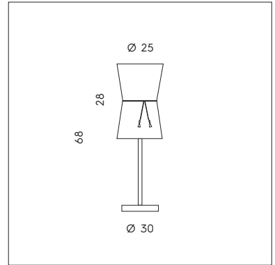
LT 1/500 1 x max 77W E27 CE
