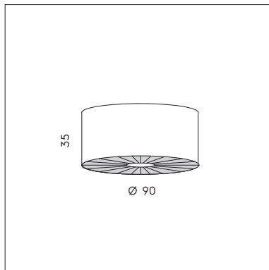
LS P/503-F 3 x max 77W E27 CE IP20 ▽
